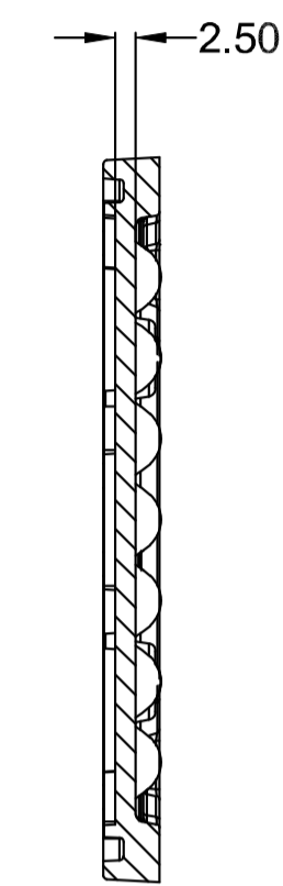
SECTION A-A
