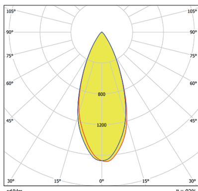
AHCOB7522D38G 38°
