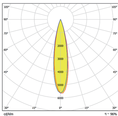
AHCOB7522D24G 24°
